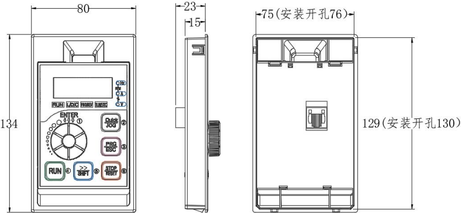
图 2-8.2 大外引键盘带托盘安装尺寸图（4T:380V 45kW以上标配大外引键盘）
