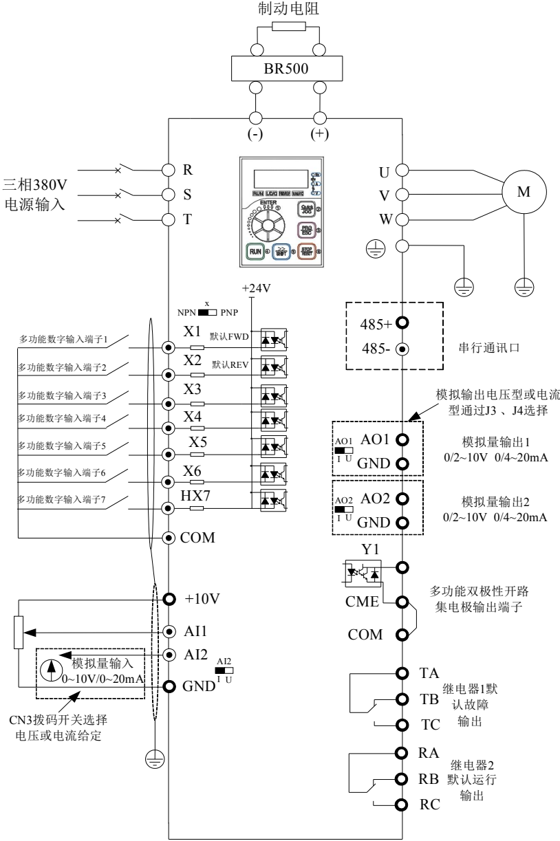
图 3-3. 三相 380V 30 ~ 55 kW (4T:380V) 变频器不带制动单元功能接线图 备注：数字输入端子 X 跳线开关出厂默认 NPN 模式（即 X 短接 COM 有效），AI2、AO1、AO2 跳线开关出厂默认电压模式。TA500/TA500S 系列 30~93kW 制动单元部分属选配功能，如有需求，订货时请说明，选配了制动单元功能的接线图参考图 3-2。
