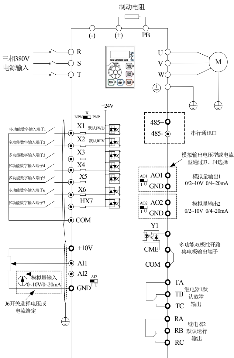
图 3-2. 三相 380V 4.0~22kW (4T:380V) 及单相 220V (3S) 5.5kW 以下(输入接 R T)变频器接线图 备注: 数字输入端子 X 跳线开关出厂默认 NPN 模式 (即 X 短接 COM 有效), AI2, A01, A02 跳线开关出厂默认电压模式
