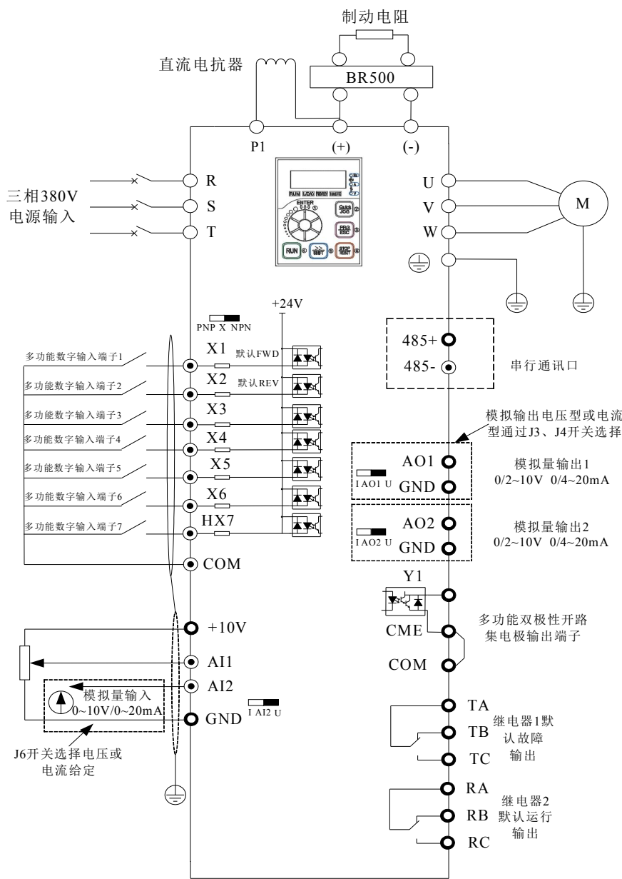
图 3-4. 三相 380V 75kW（4T:380V）及以上三相变频器接线图 备注：数字输入端子 X 跳线开关出厂默认 NPN 模式（即 X 短接 COM 有效），AI2, AO1, AO2 跳线开关出厂默认电压模式。TA500/TA500S（4T:380V）75~132kW 外置直流电抗器选配，160kW(含 160kW) 以上内置直流电抗器标配。
