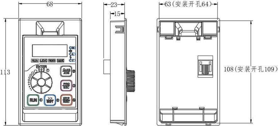
图 2-8.1 小外引键盘带托盘安装尺寸图（4T:380V 37kW以下标配小外引键盘）
