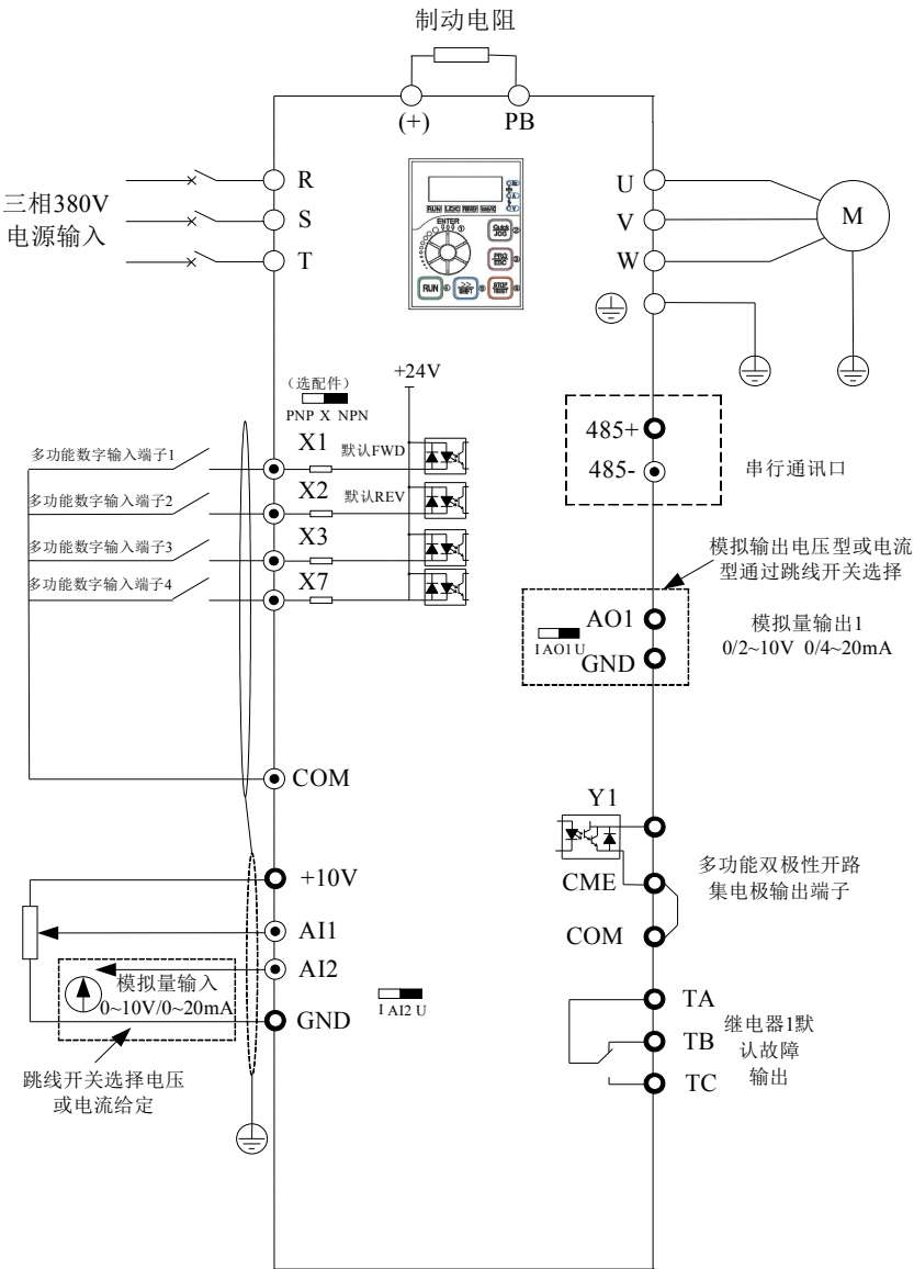
图3-1. 三相380V 2.2kW (4T:380V) 及单相220V (3S) 1.5kW(输入接L N或R T) 以下变频器接线图 备注：数字输入端子X跳线开关出厂默认NPN模式（即X短接COM有效），PNP模式为选配功能，三相380V 2.2 kW 及单相220V 1.5 kW 以下如需选配PNP模式，订货时请说明。AI2, AO1跳线开关出厂默认电压模式。
