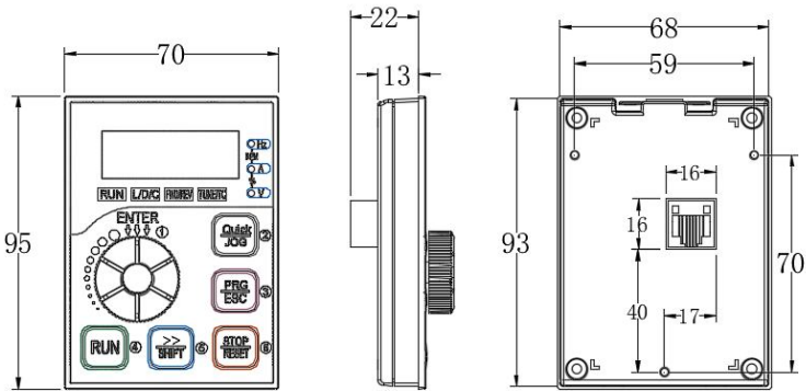
图 2-9.2 大外引键盘不带托盘安装尺寸图（4T:380V 45kW以上标配大外引键盘）
