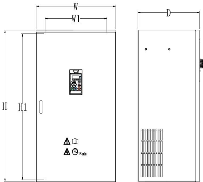
图 2-6. 380V 160kW 以上变频器外型尺寸及安装尺寸示意图
